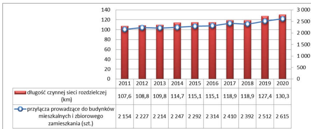
Wykres 5. Długość czynnej sieci wodociągowej w km oraz liczba przyłączy
